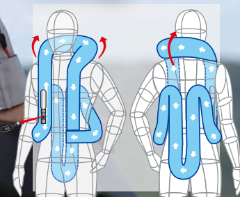
エアバッグ構造
