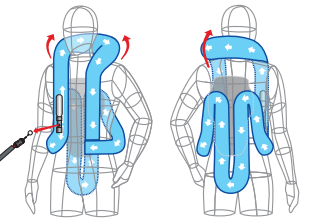
エアバッグ展開図
