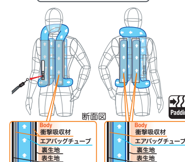
エアバッグ展開図
